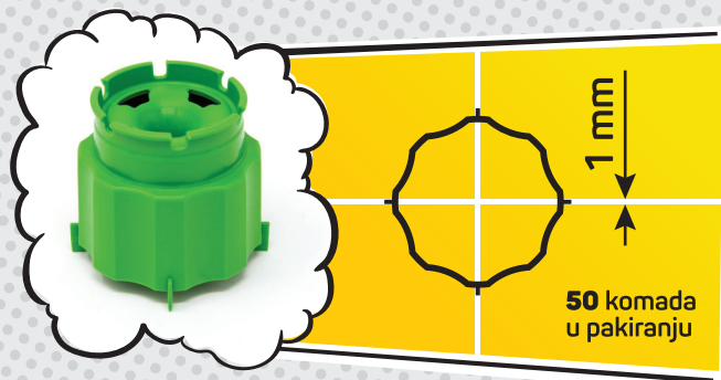
KRIŽNI (SL BASE) SLBC 1 šifra artikla: 004410
