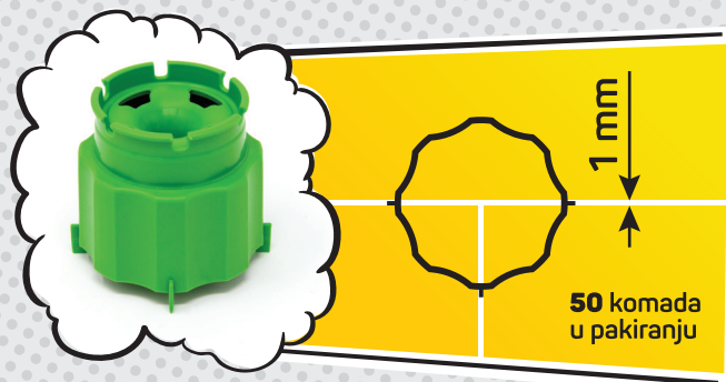
T-OBLIK (SL BASE) SLBT 1 šifra artikla: 004408
